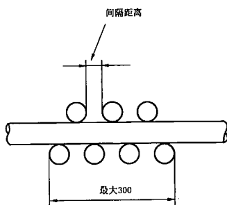
图 1 安装在标准钢梯两侧的电线的典型排列和间隔(A F/R 类)
